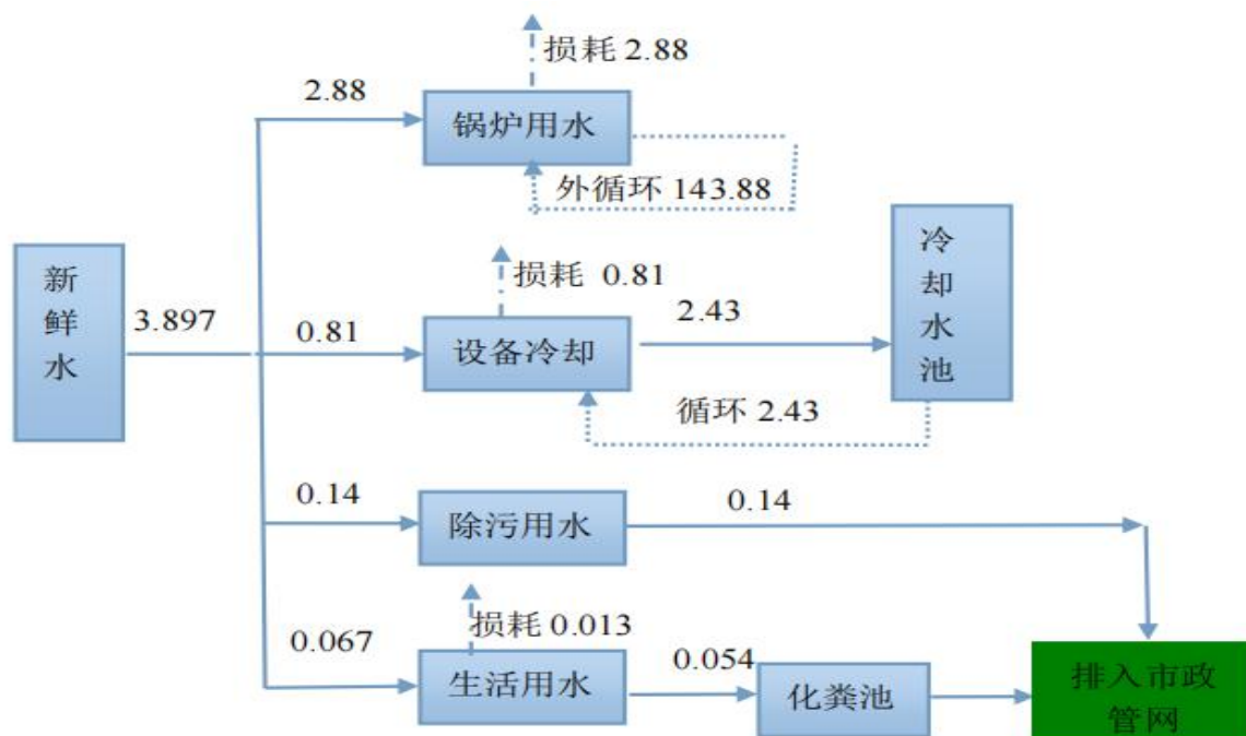
项目给排水平衡图 单位 m 3 /h
